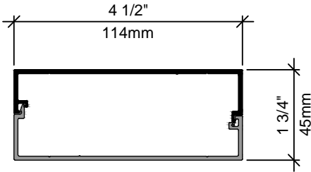
SS10 OUTRIGGER
