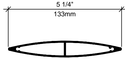
SS40 LOUVER
