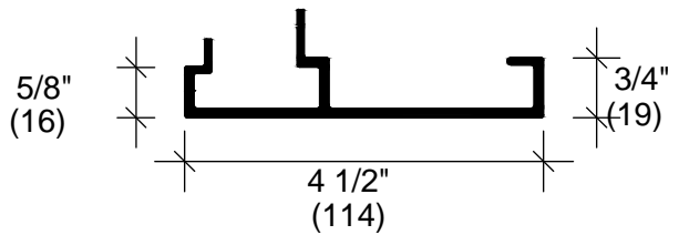
C2515 DOOR ADAPTER
